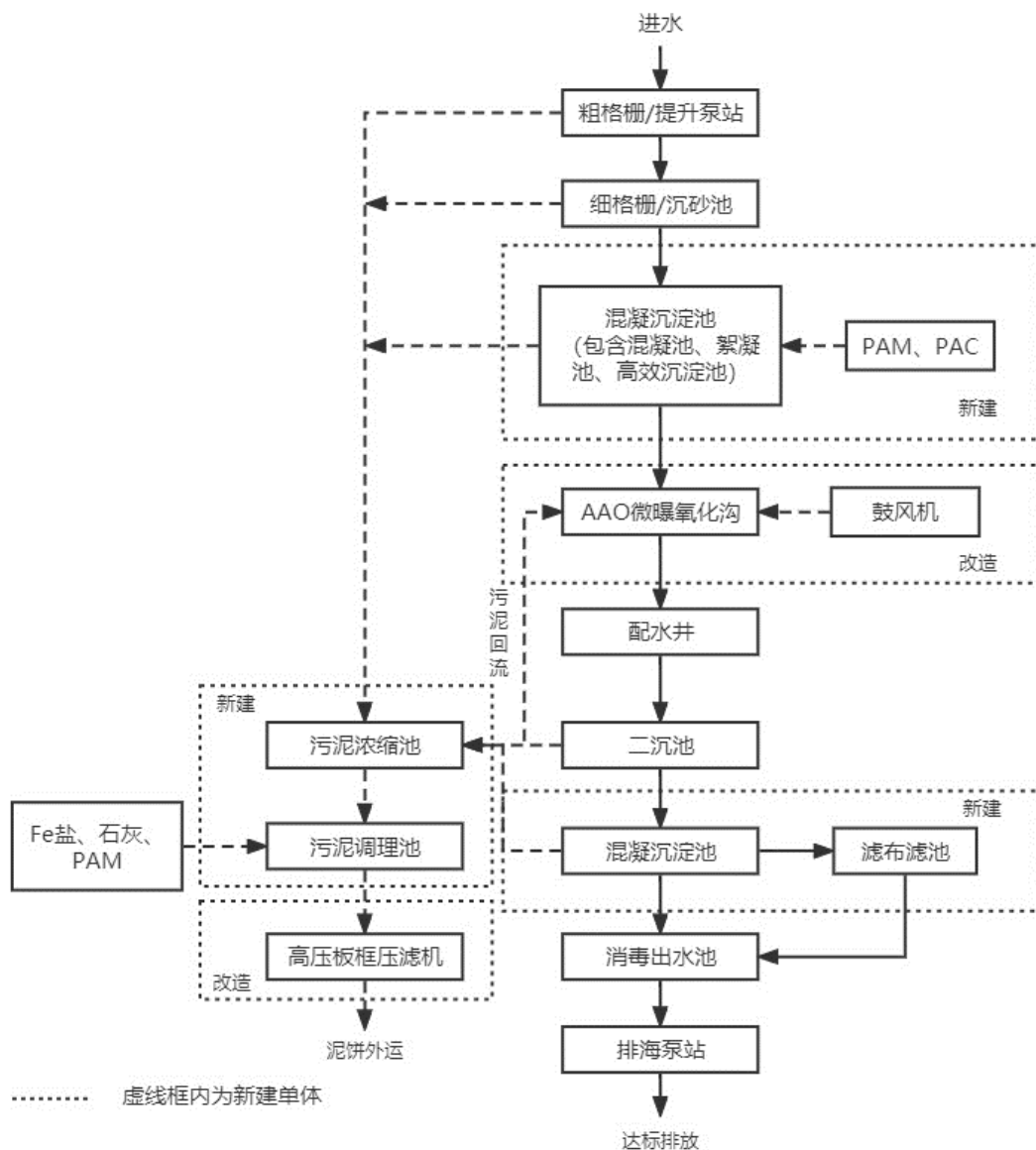
图 2.3-2 改造 12500m 3 /d 污水处理厂总工艺流程图
