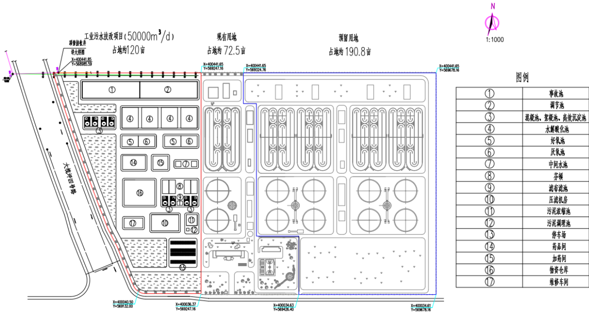
图 2.2-1 总平面布置
