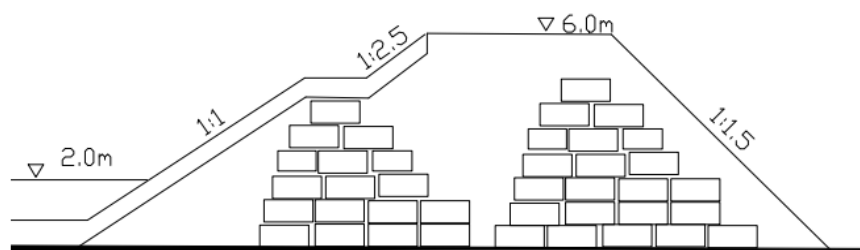
图 2.4-1 围堰断面构造示意图（单位：米，1985 国家高程基准）
