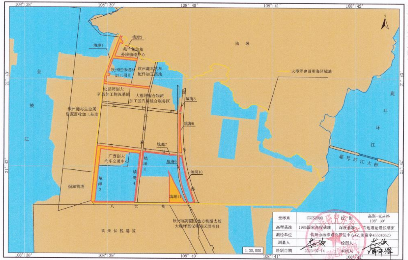
大榄坪装备制造产业园基础设施配套项目平面布置图
