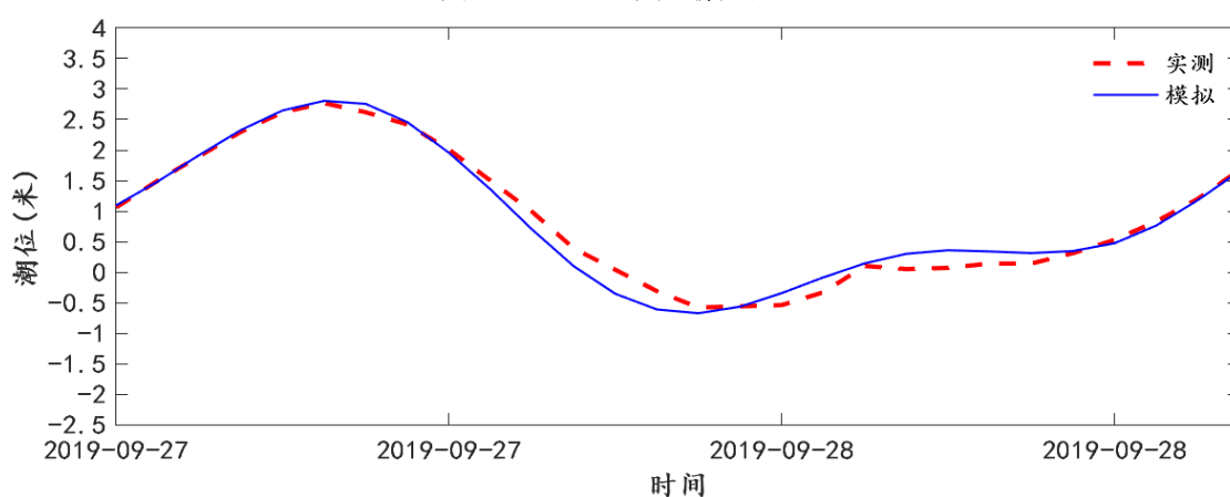
图 4.3-4 CW2 站位潮位验证
