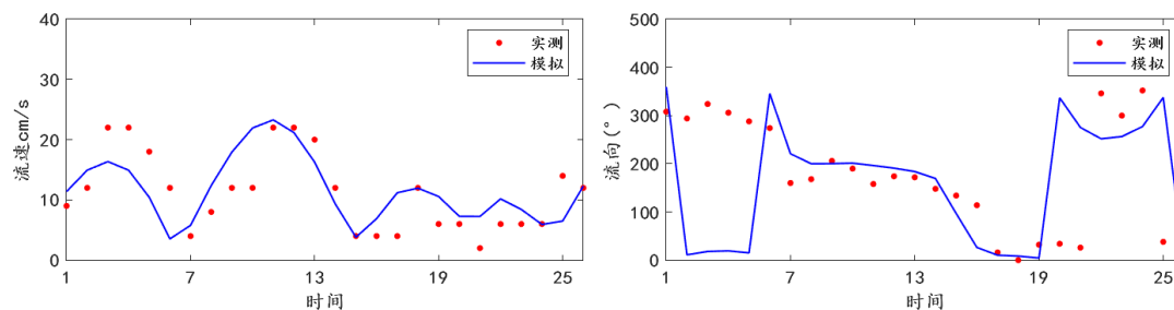
图 4.3-8 CL3 流速流向验证
