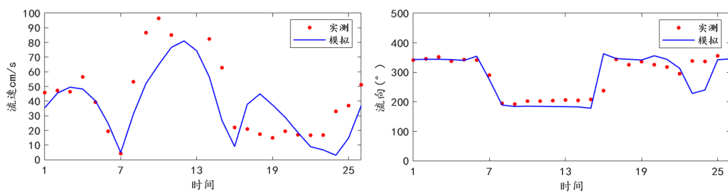
图 4.3-6 CL1 流速流向验证
