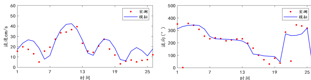
图 4.3-2 CL6 流速流向验证
