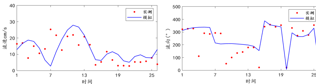
图 4.3-9 CL4 流速流向验证
