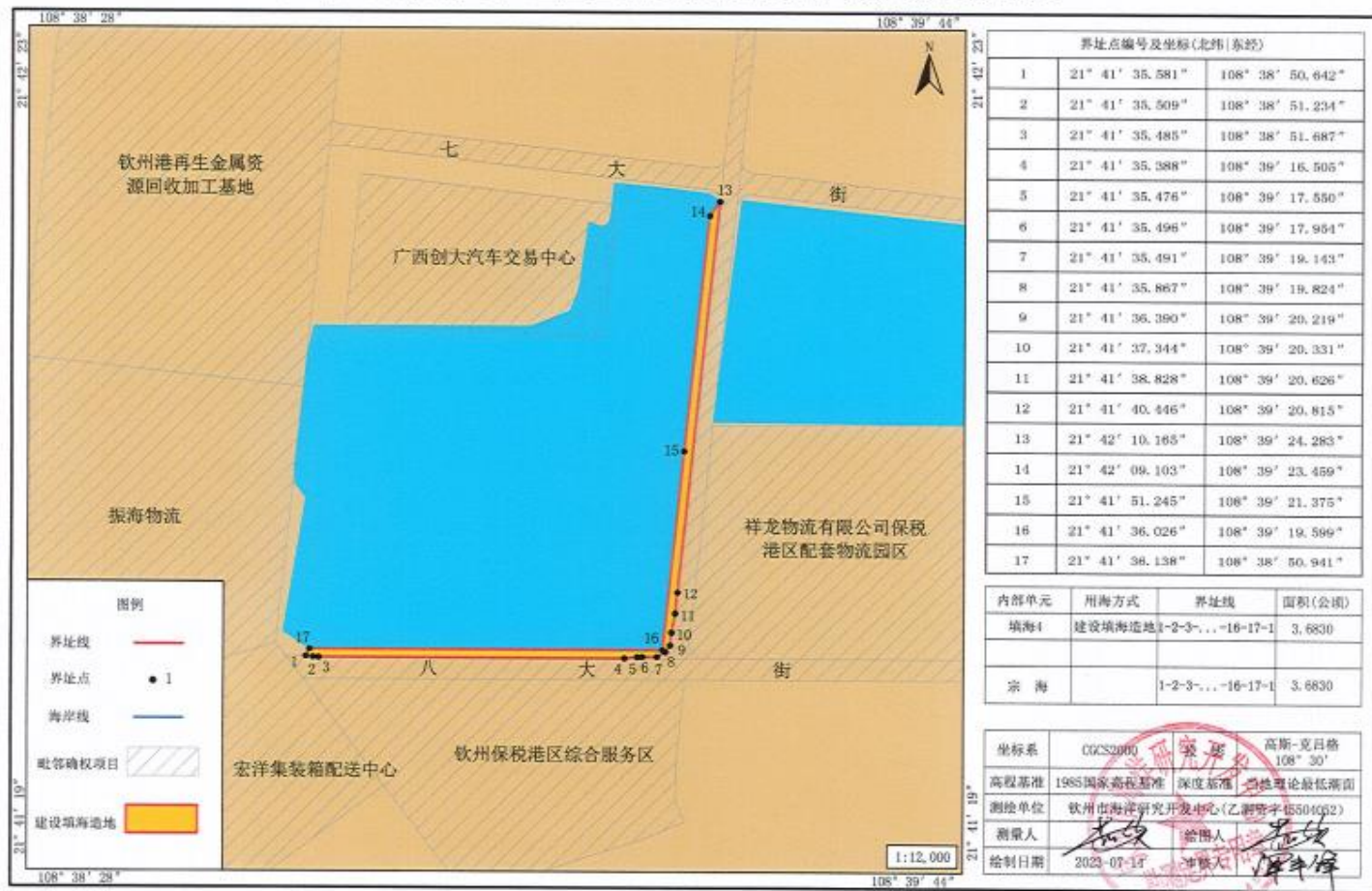
大榄坪装备制造产业园基础设施配套项目填海4宗海界址图
