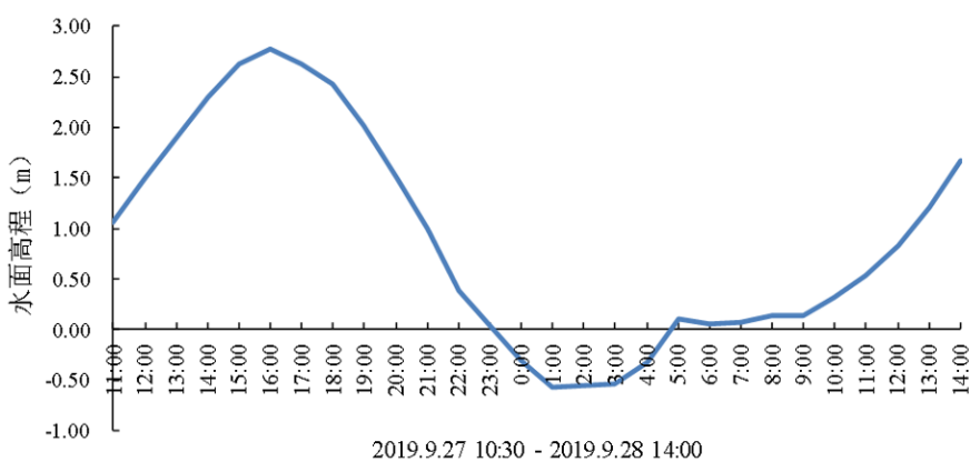
图 3.2-5 企沙临时验潮站 (CW3) 潮位曲线 (85 高程)
