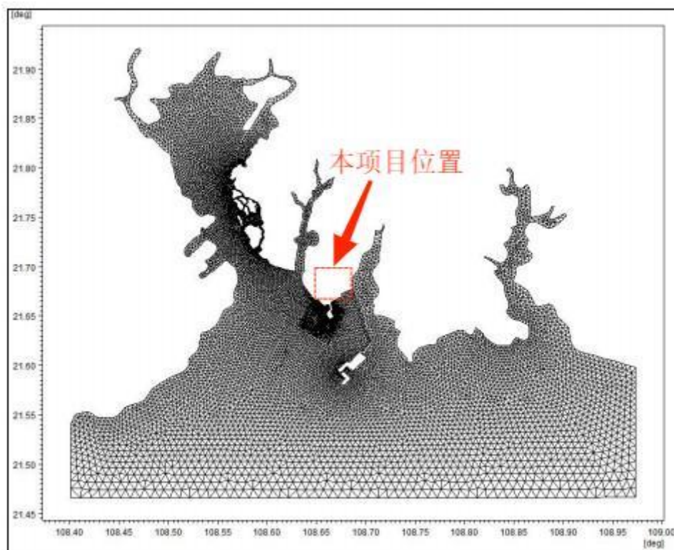
图 4.3-1 模型计算区域和网格分布
