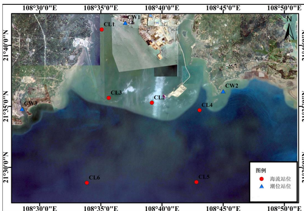
图 4.3-2 潮位和海流实测站位分布图
