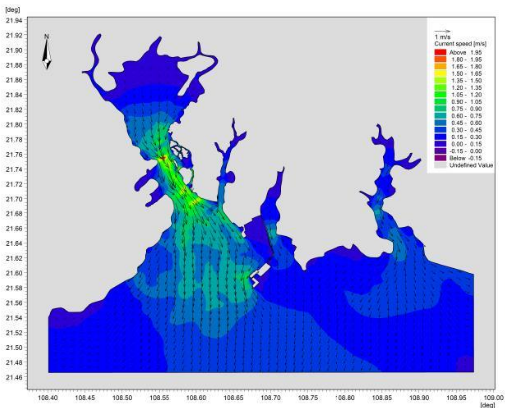
图 4.3-13 钦州湾现有岸线数值模型大潮时涨急时刻流场
