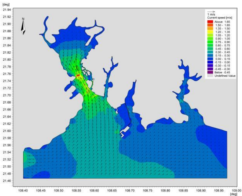
图 4.3-12 钦州湾现有岸线数值模型大潮时涨急时刻流场
