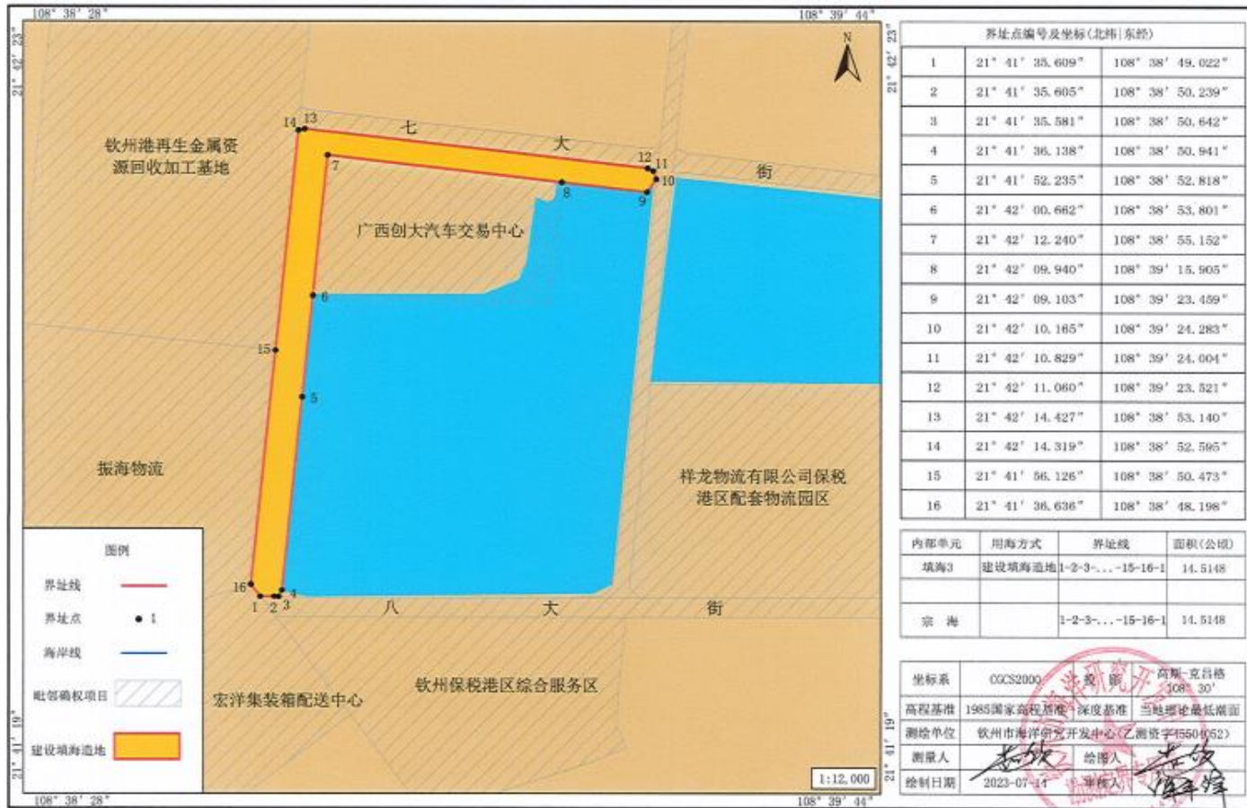
大榄坪装备制造产业园基础设施配套项目填海3宗海界址图
