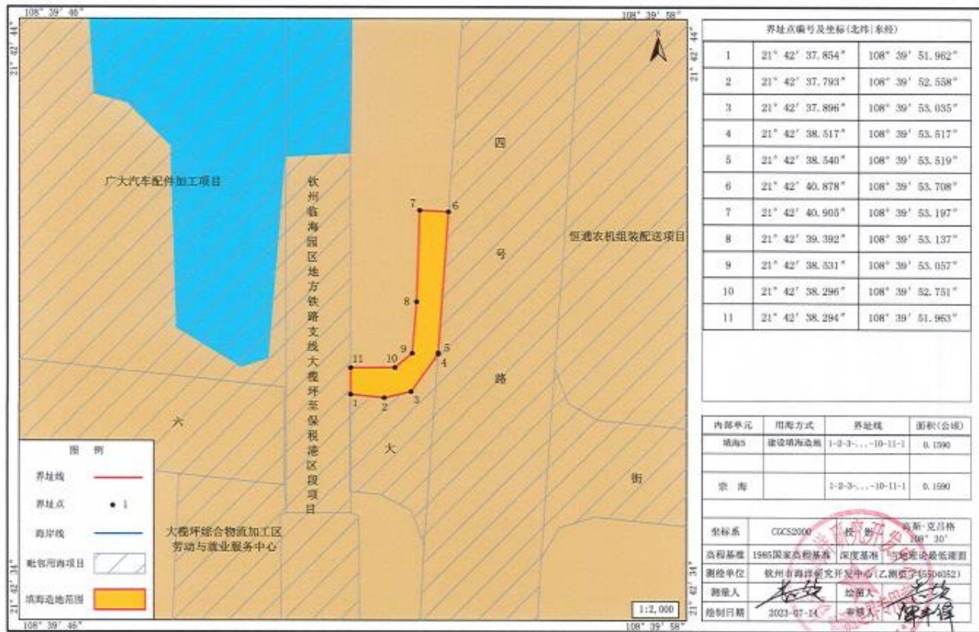
大榄坪装备制造产业园基础设施配套项目填海5宗海界址图
