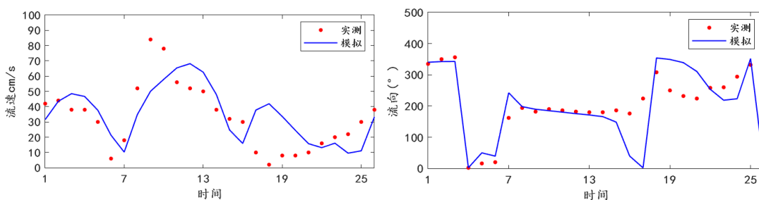
图 4.3-7 CL2 流速流向验证
