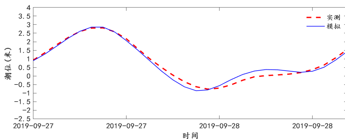
图 4.3-3 CW1 站位潮位验证
