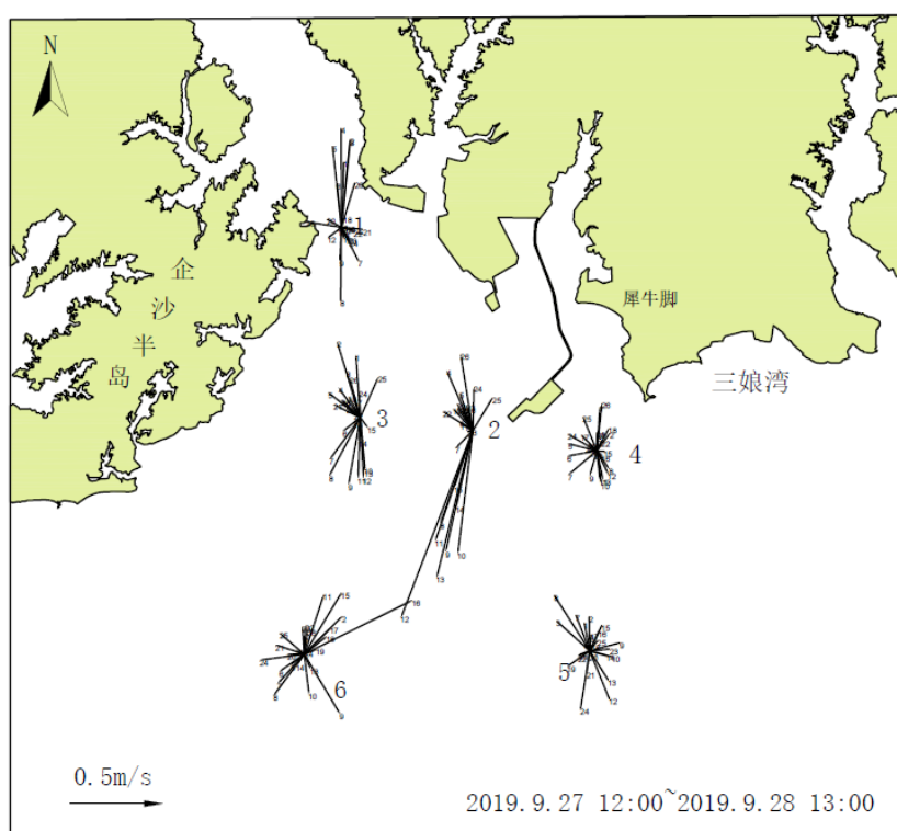
图 3.2-7 2019 年 9 月海流观测矢量图（底层）
