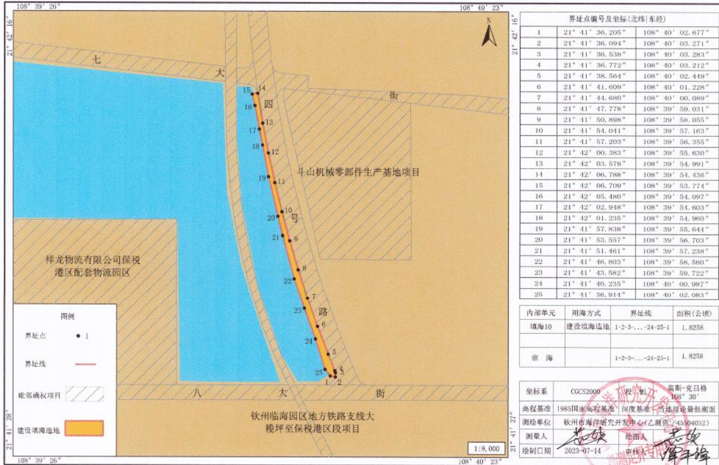
大榄坪装备制造产业园基础设施配套项目填海10宗海界址图
