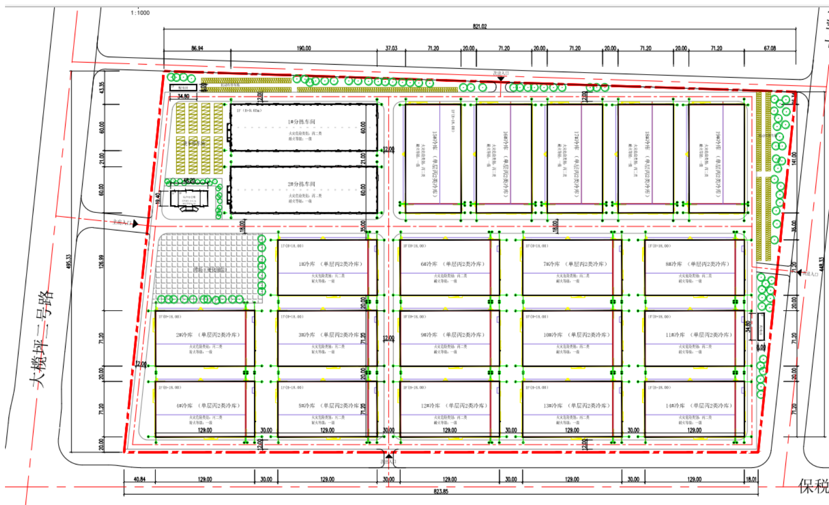
图 7.2.2-1 平面布置推荐方案 (方案一)
