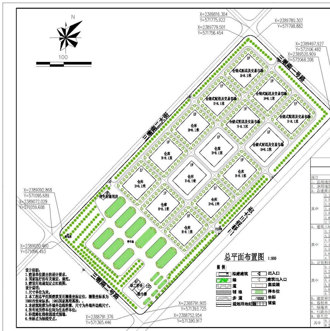
图 1.1-2 项目总平面布置示意图
