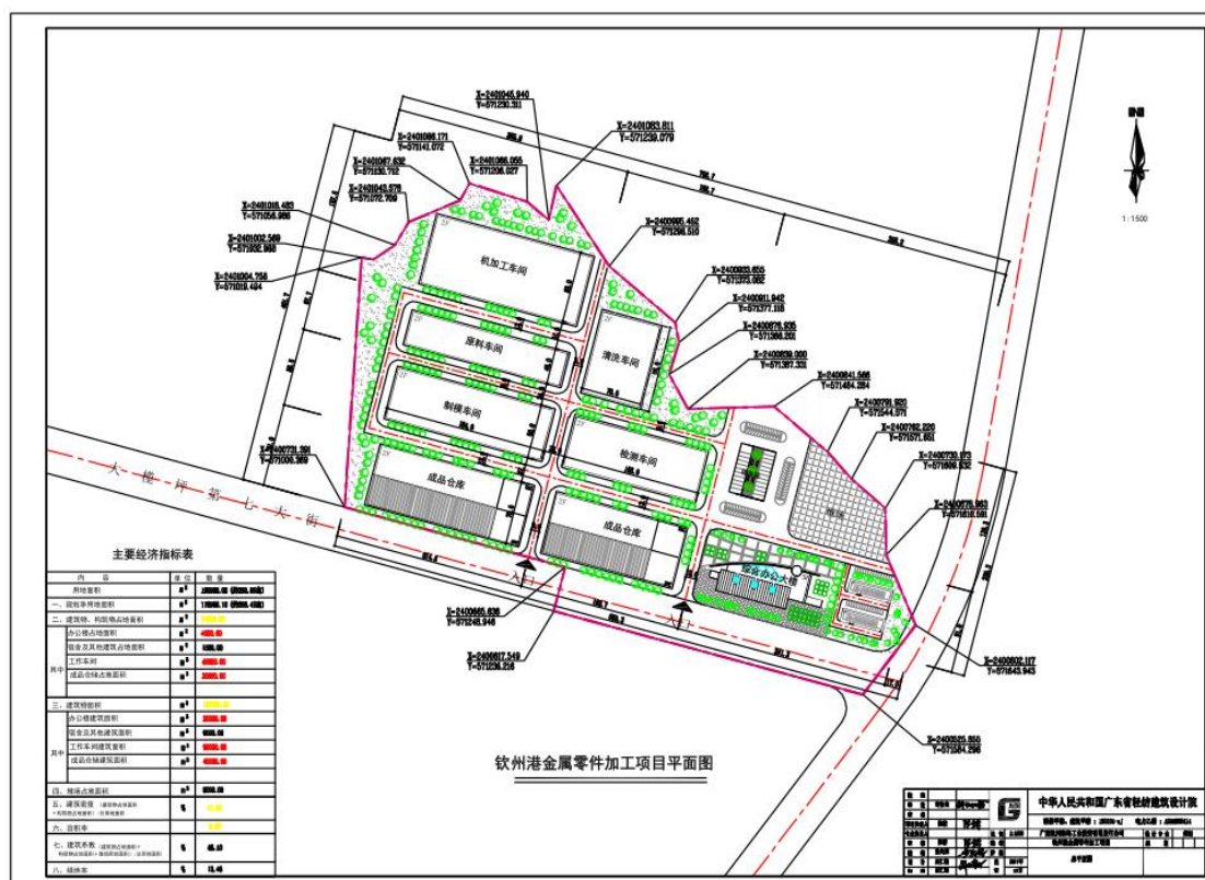
图 1.2-2b 拟建工程平面布置图
