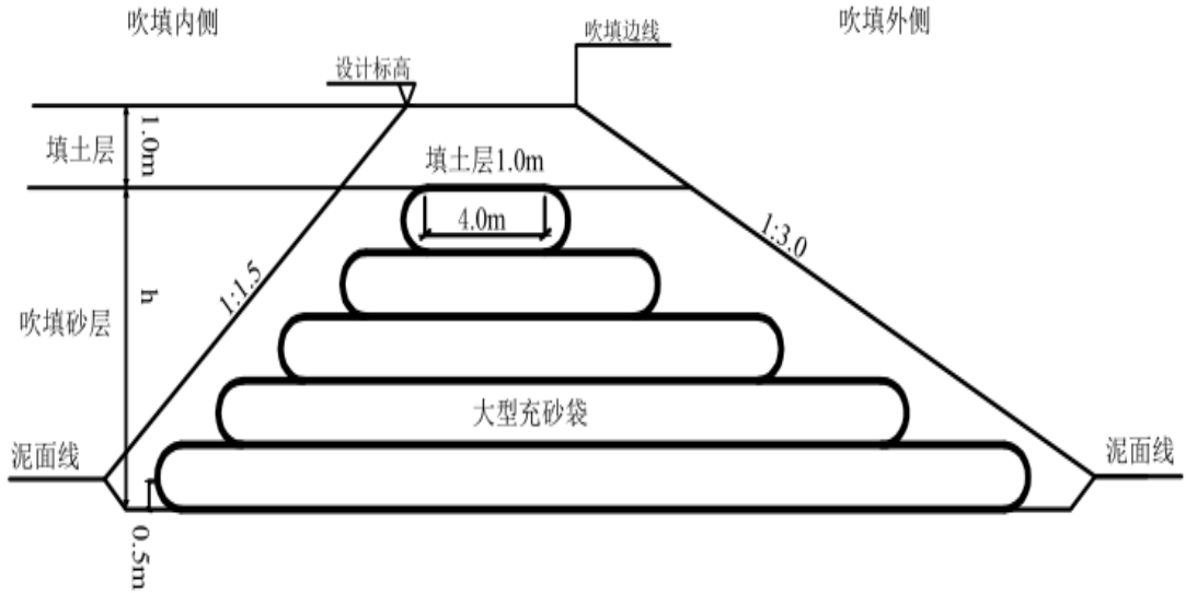
图 1.2-3 围埝结构断面图
